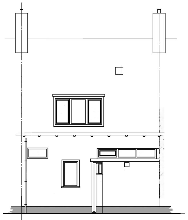
ACHTERGEVEL
