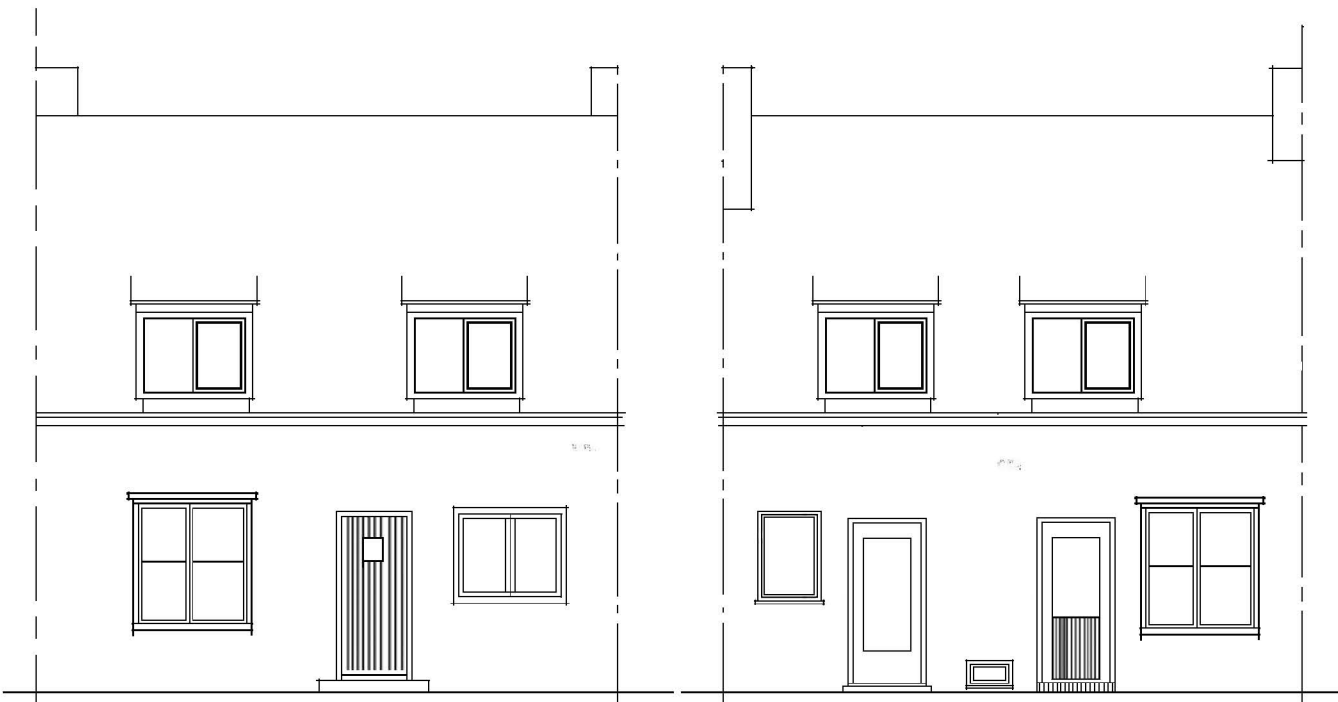
VOORGEVEL (noord orientering)
