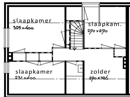
VERDIEPING
