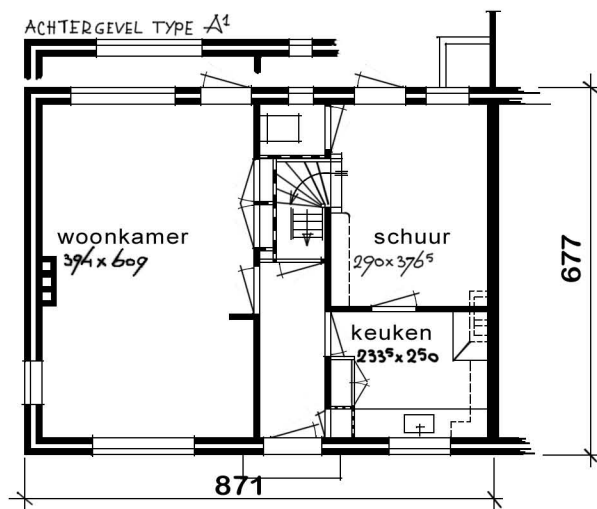
BEGANE GROND
