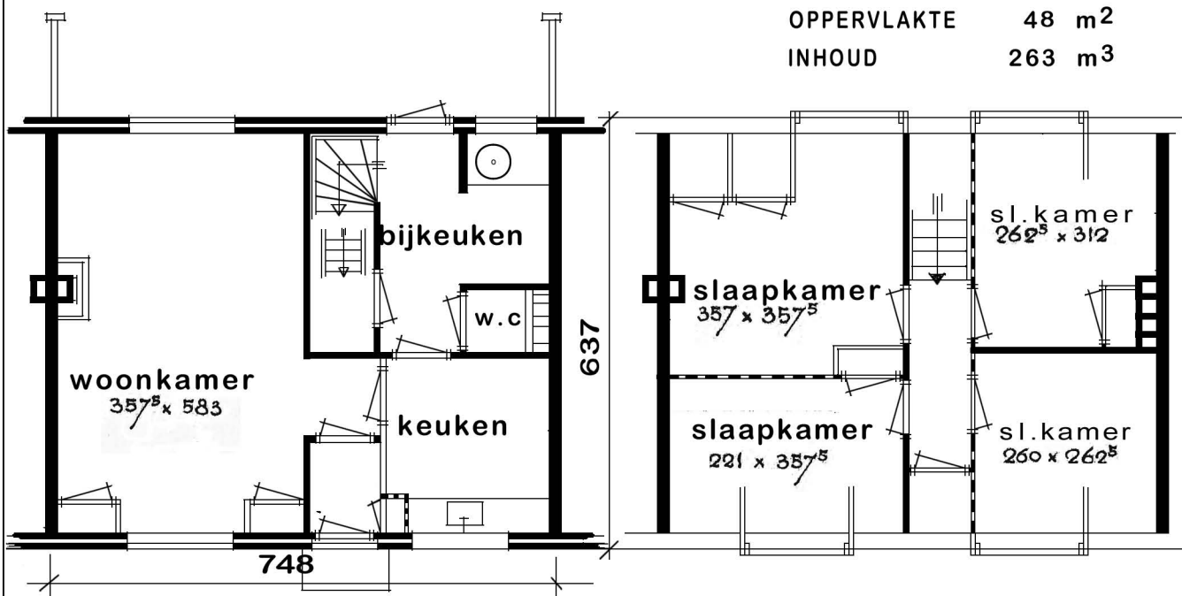
BEGANE GROND
