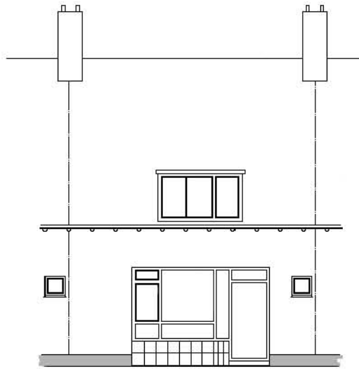
VOORGEVEL.
