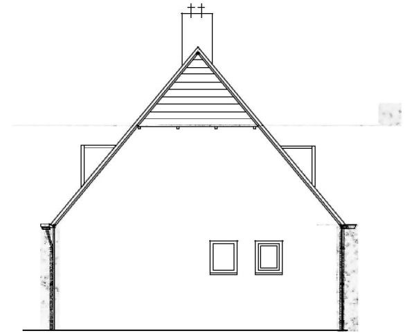
ZUGEVEL beklede topgevel alleen voor C 2
