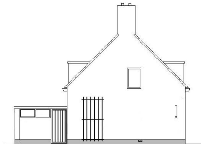
ZIJGEVEL
