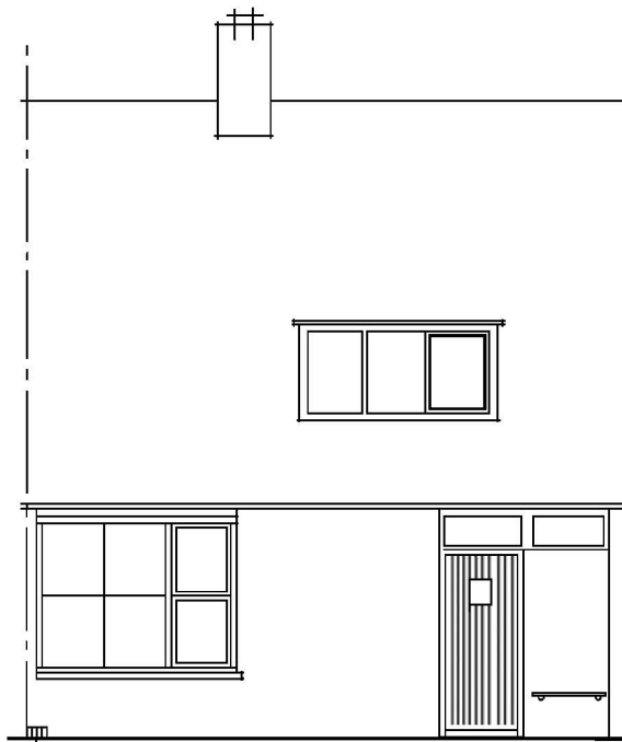
VOORGEVEL TYPE C
