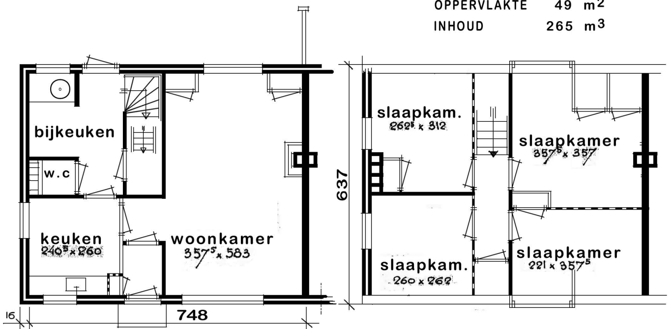
BEGANE GROND
