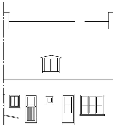
ACHTERGEVEL
