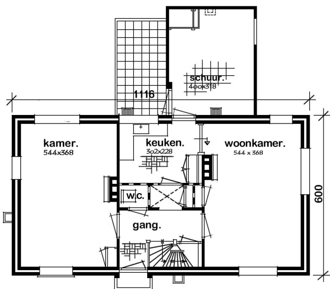
BEGANE GROND
