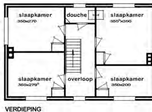
VERDIEPING
