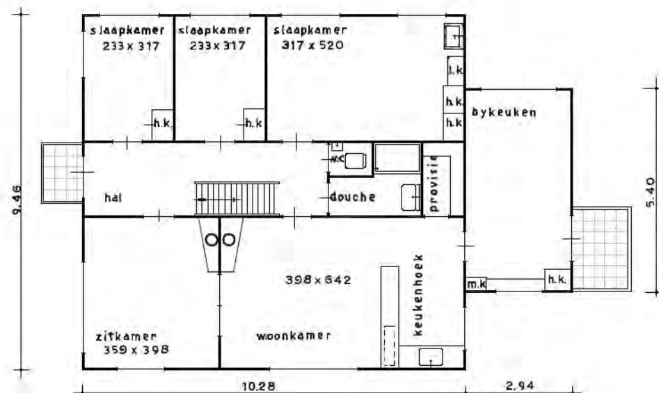
BEGANEGROND.
