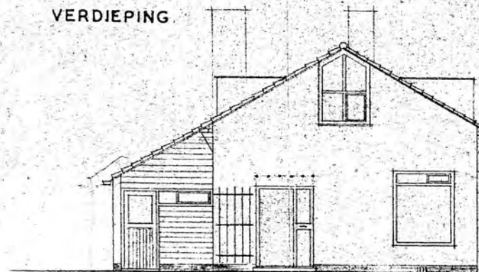
ZIJGEVEL
