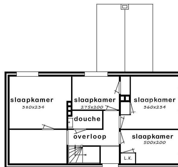
VERDIEPING
