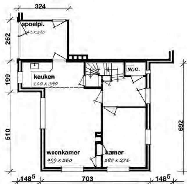
BEGANE GROND
