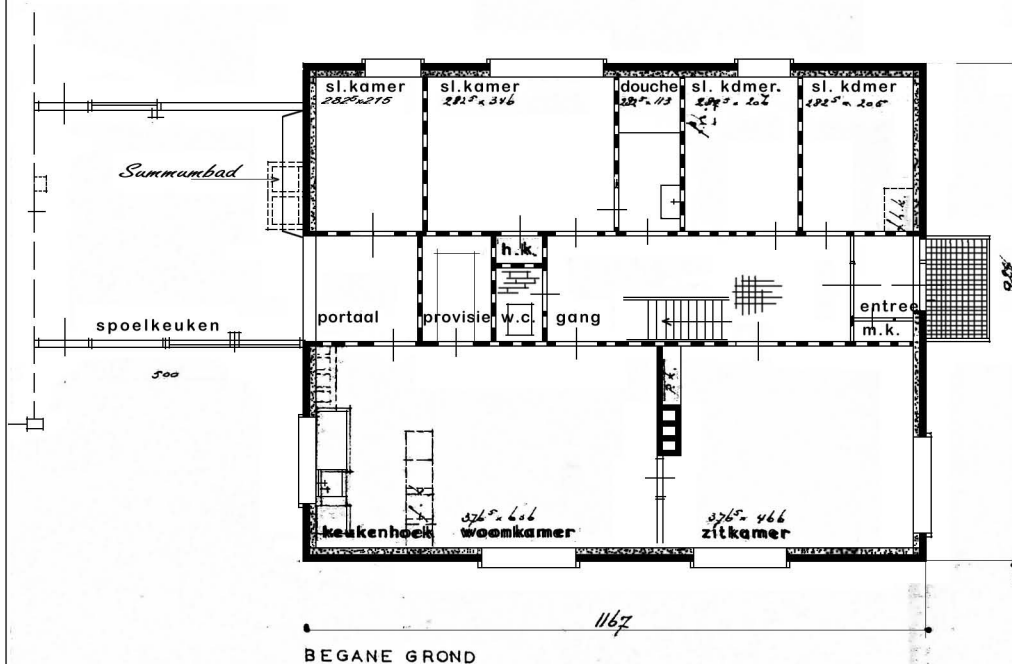
BEGANE GROND
