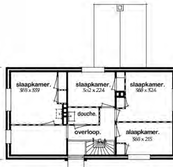
VERDIEPING
