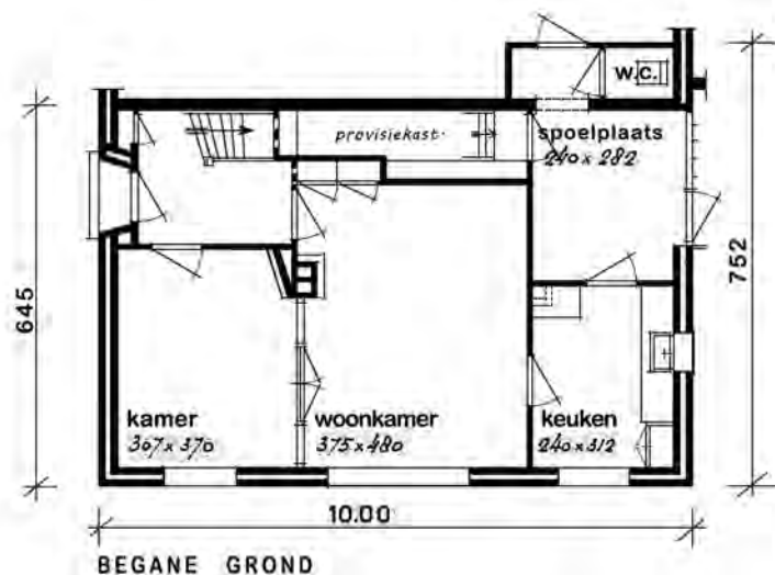
BEGANE GROND
