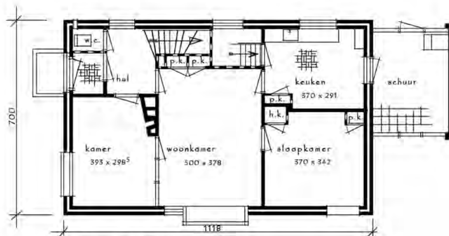
BEGANE GROND
