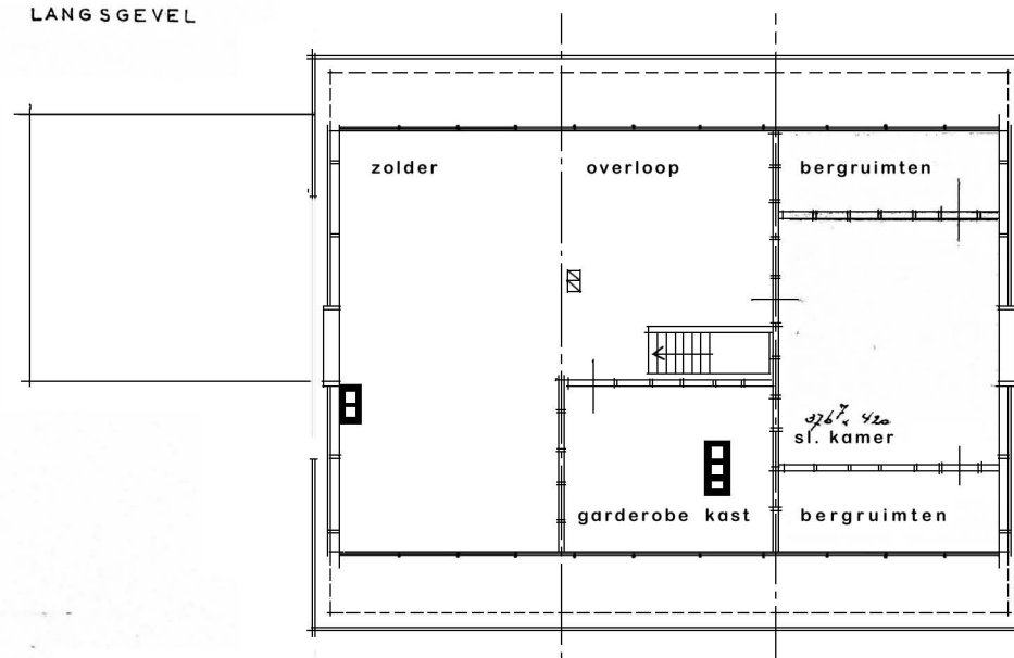
VERDIEPING
