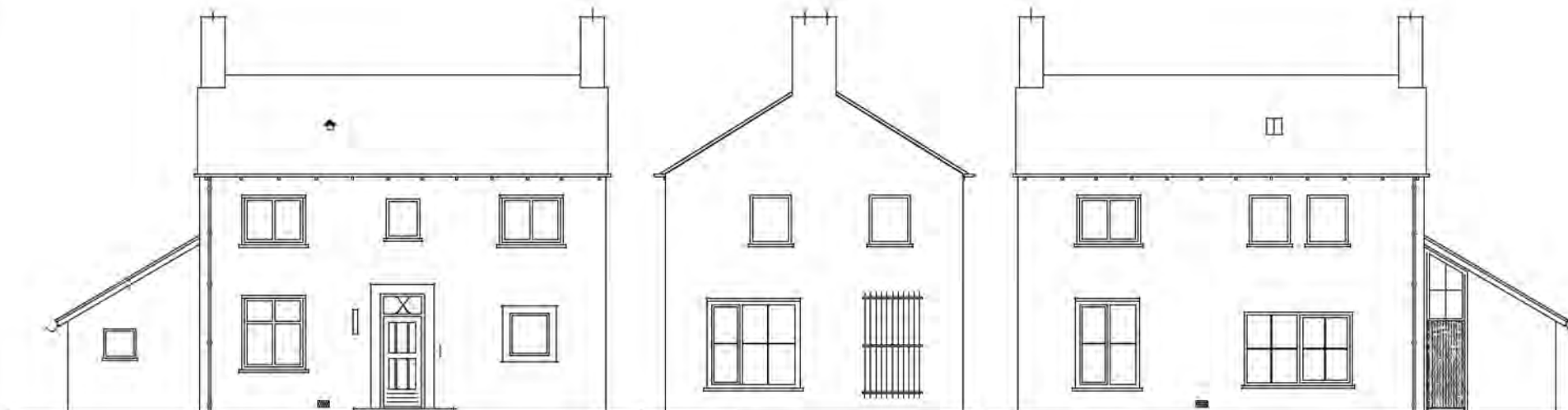
VOORGEVEL
