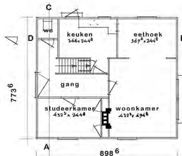
BEGANE GROND
