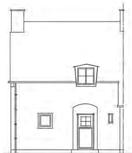
RECHTER ZUGEVEL
