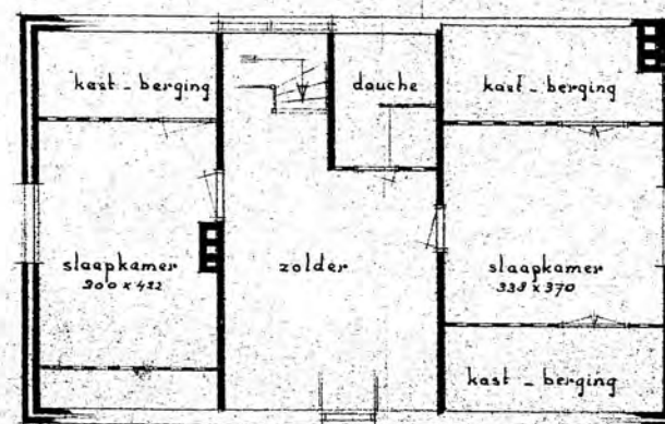
VERDIEPING
