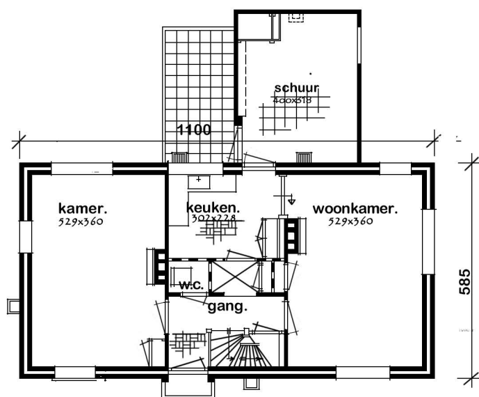
BEGANE GROND
