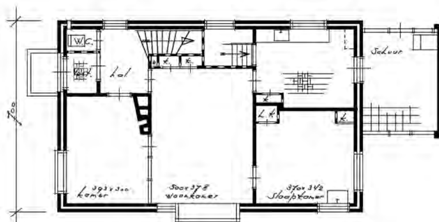
BEGANE GROND
