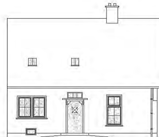
LINKERZIJGEVEL
