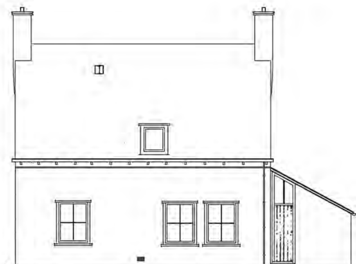
ACHTERGEVEL
