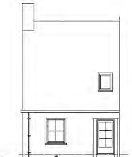
R - ZIJGEVEL
