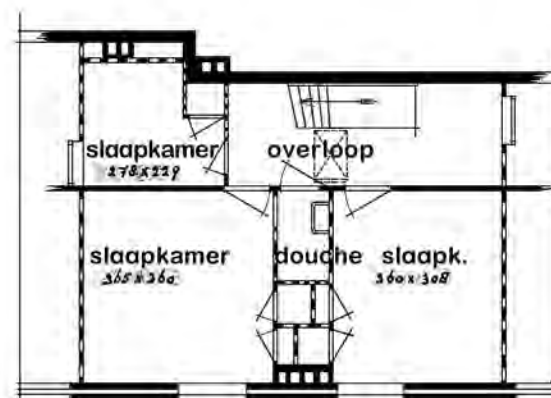
VERDIEPING
