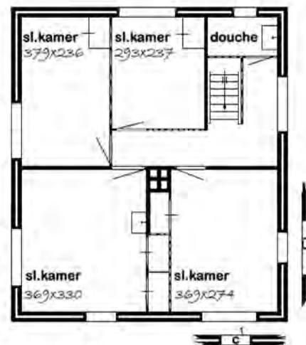
VERDIEPING
