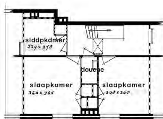
VERDIEPING
