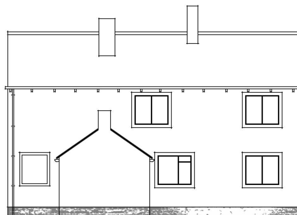
ACHTERGEVEL
