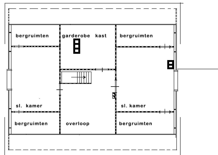
VERDIEPING
