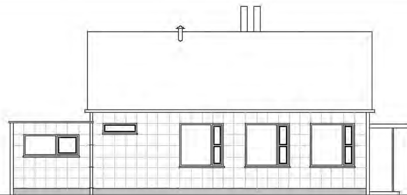
LINKERZUGEVEL.
