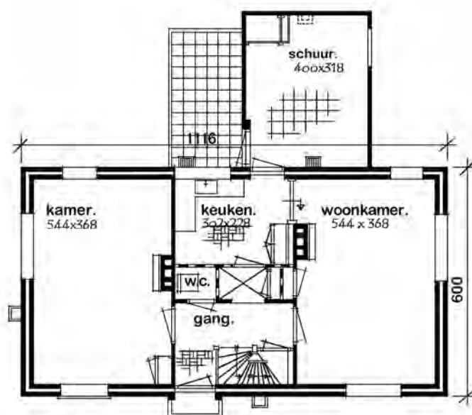
BEGANE GROND
