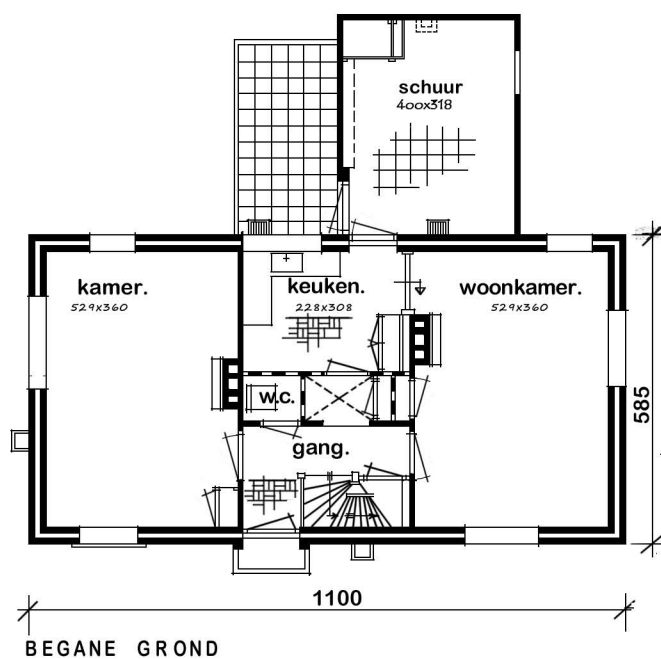
BEGANE GROND
