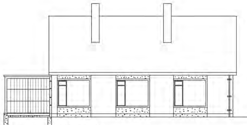
LANGSGEVEL
