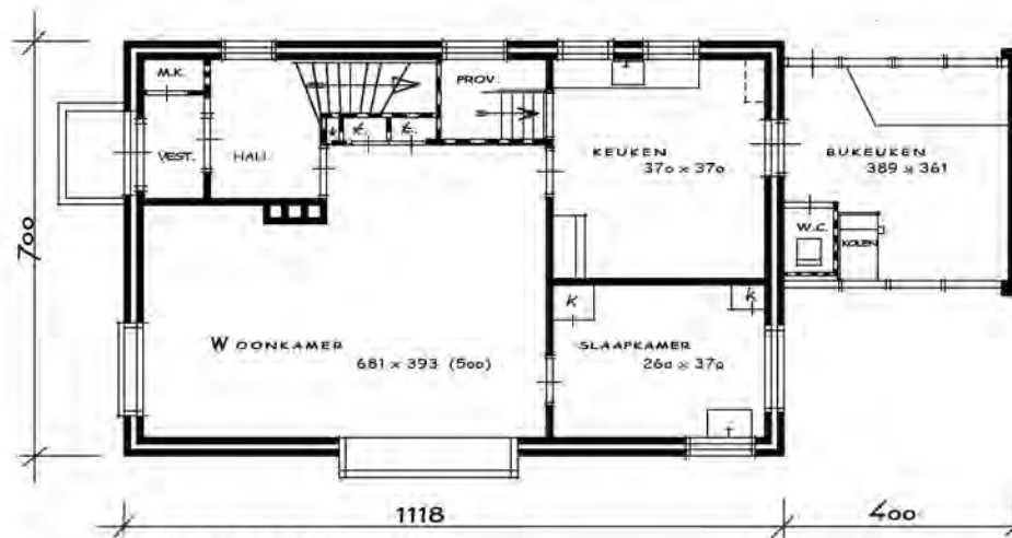
BEGANEGROND
