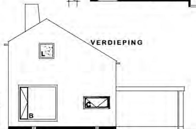
VOORAANZICHT
