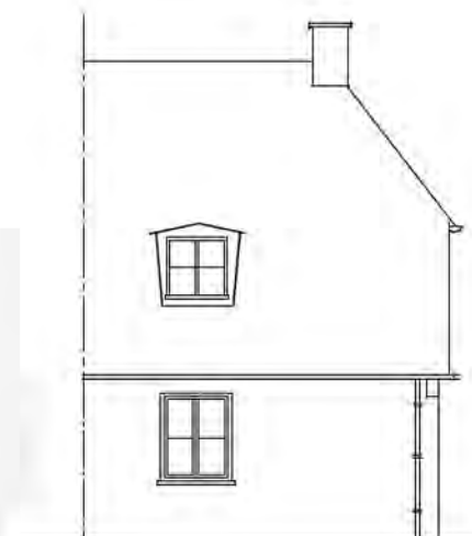
L. ZIJGEVEL
