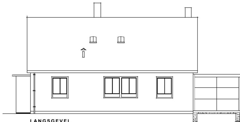
LANGSGEVEL
