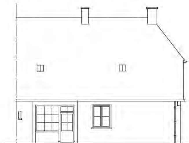
L. ZUGEVEL
