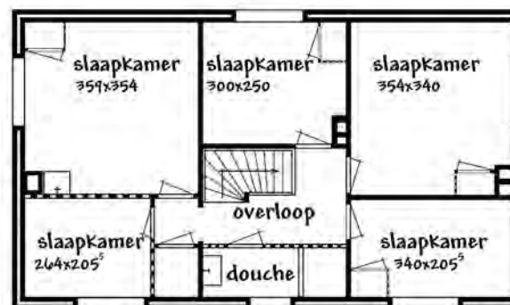
VERDIEPING
