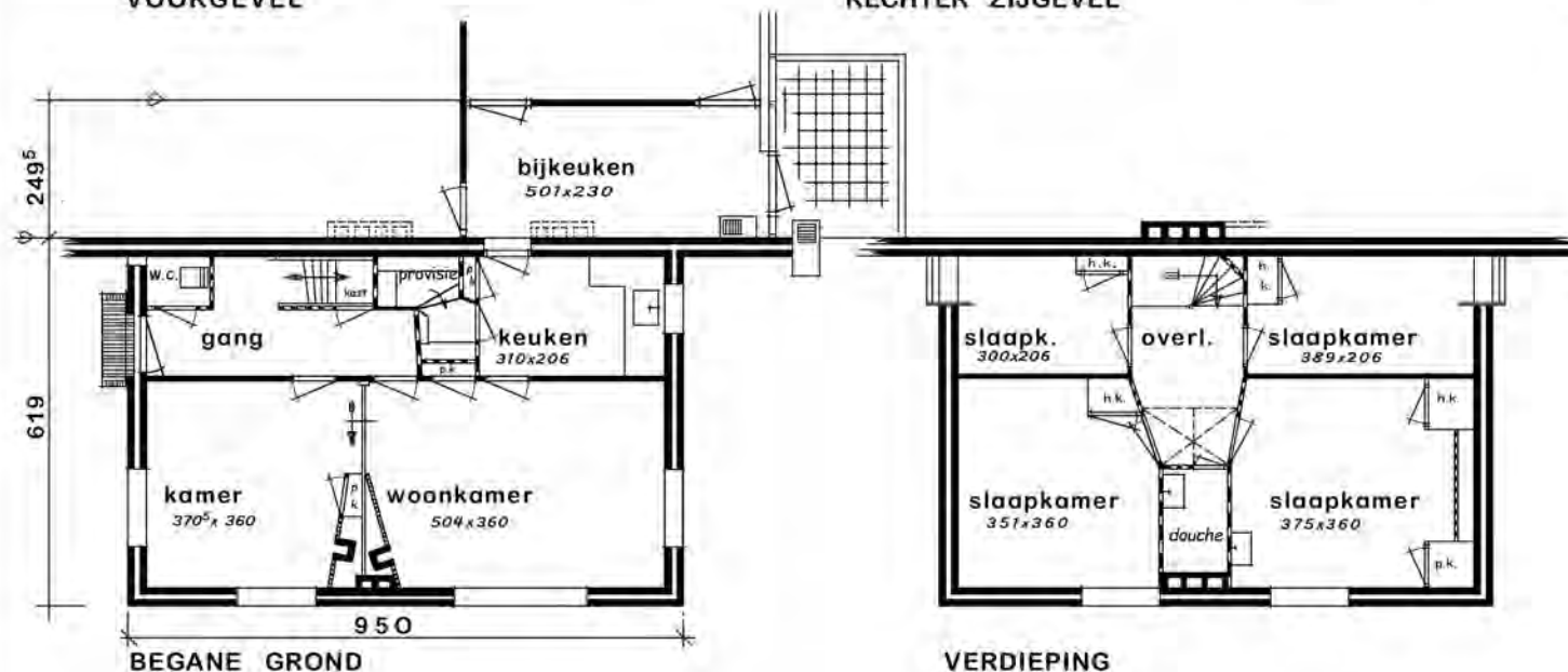
BEGANE GROND
