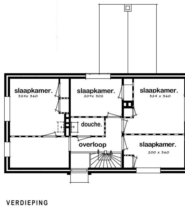
VERDIEPING
