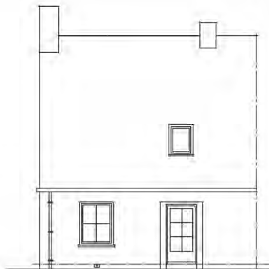
RECHTER ZIJGEVEL
