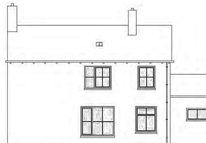
ACHTERGEVEL
